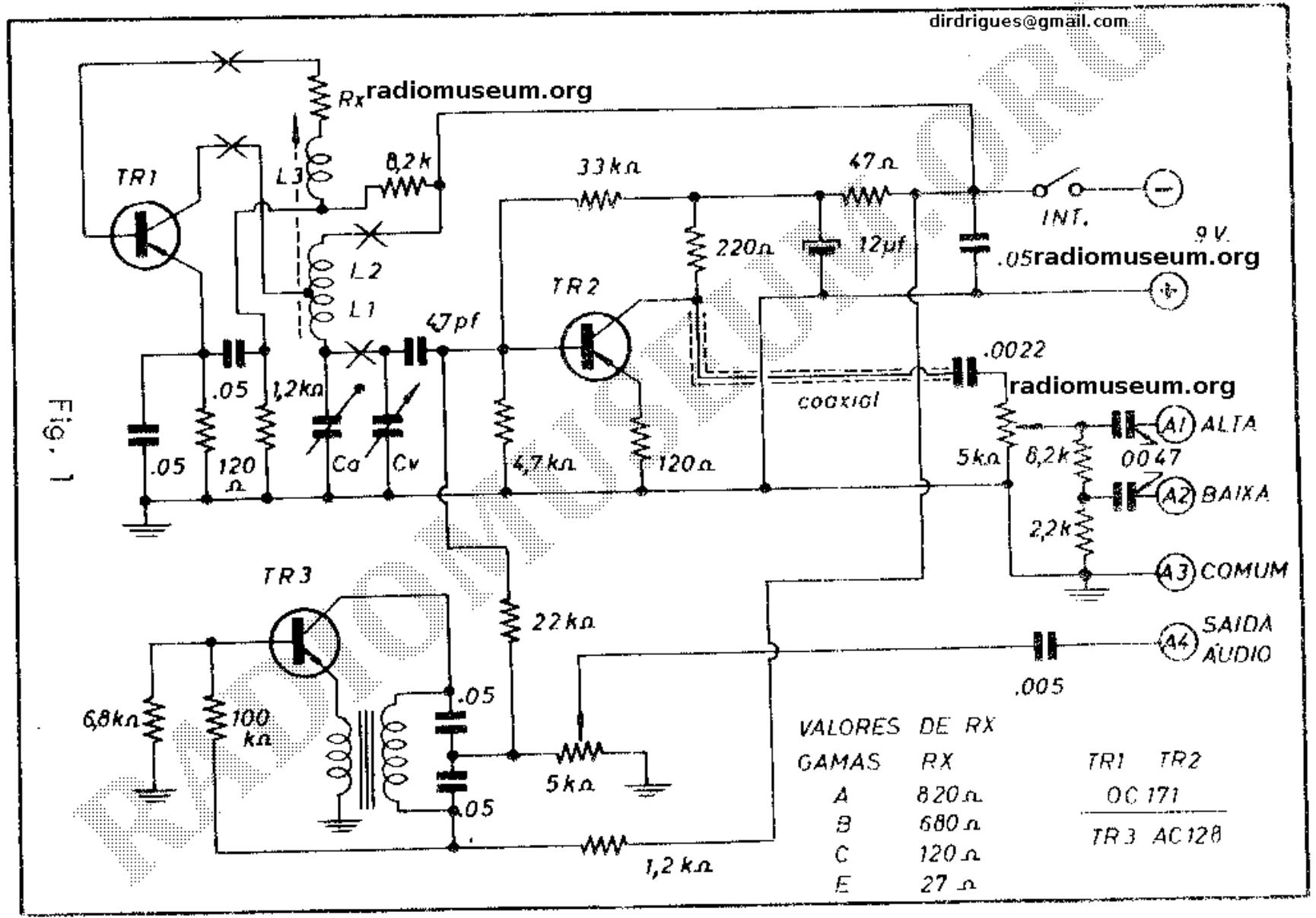
Esquema geral do oscilador de R.F. Mod. O4
