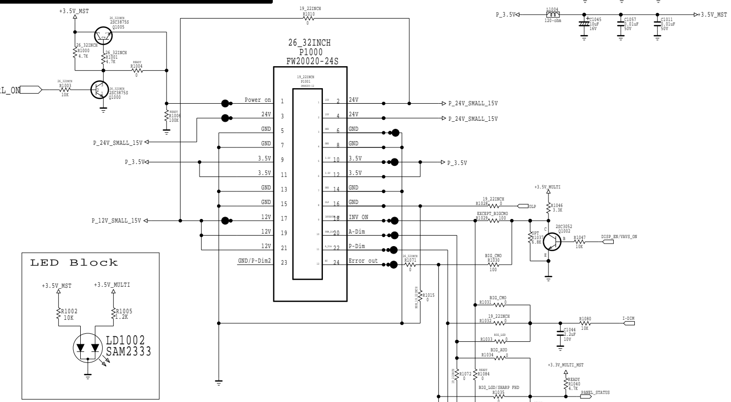
<OS MODULE PIN MAP>
